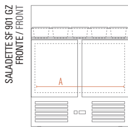
SALADETTE SF 901 GZ ESEMPIO CONFIGURAZIONE BACINELLE GN EXAMPLE GN TRAY CONFIGURATION
