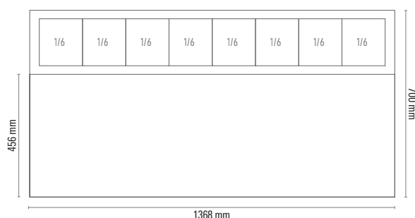
SALADETTE SF 903 GZ ESEMPIO CONFIGURAZIONE BACINELLE GN EXAMPLE GN TRAY CONFIGURATION
