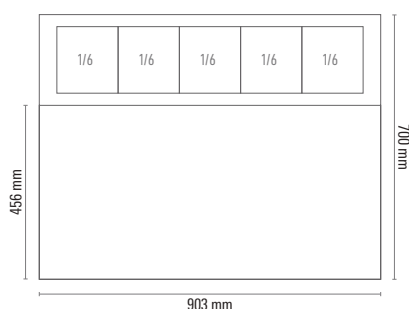
SALADETTE SF 901 GZ ESEMPIO CONFIGURAZIONE BACINELLE GN EXAMPLE GN TRAY CONFIGURATION
