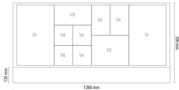
SALADETTE SF 903 G ESEMPIO CONFIGURAZIONE BACINELLE GN EXAMPLE GN TRAY CONFIGURATION
